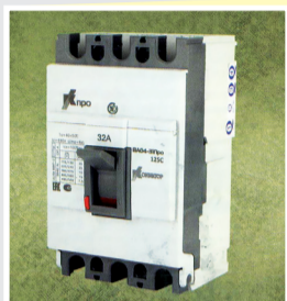
Выключатель автоматический. ТМ «Контактор». Серия ВА04-31ПРО
